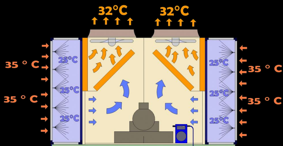
SYSTÉM PŘEDCHLAZENÍ JE V PROVOZU
